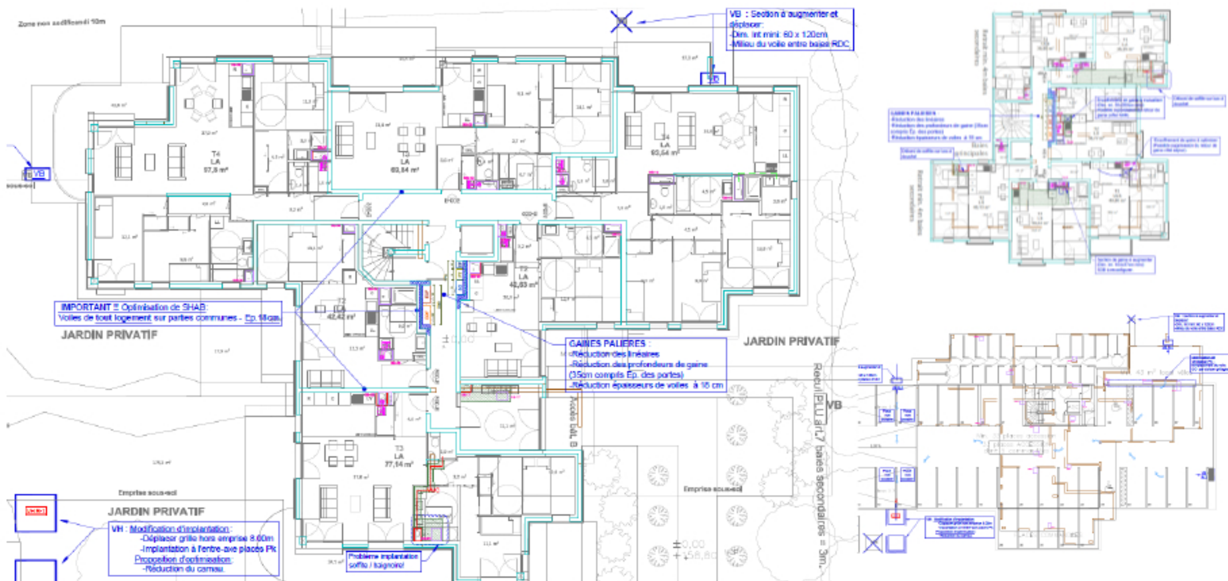
Pré étude Fluides sur plan de niveau avant projet architecte:
